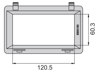
挖孔尺寸图
