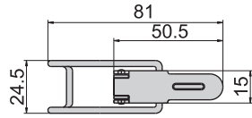
CKC-1037 CKC-37
