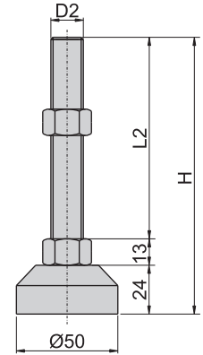
S50 无防滑橡胶盘垫
