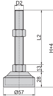
KMS50 配加防滑橡胶盘垫
